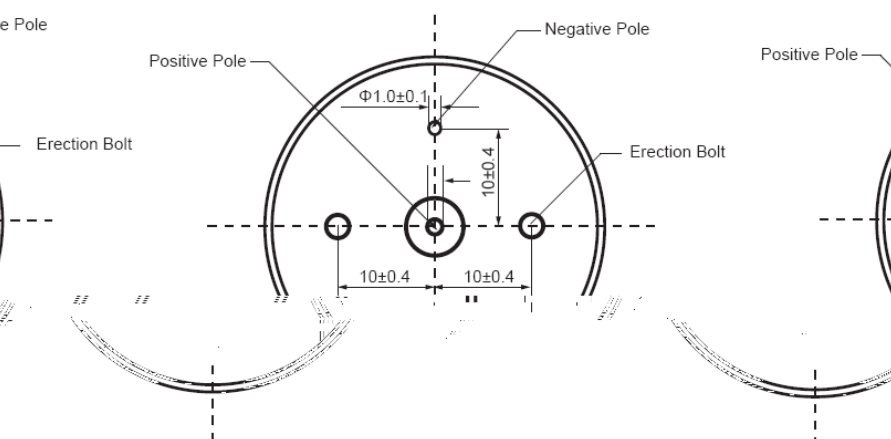
THC2W Φ36x12/16 outline (B) Unit:mm
